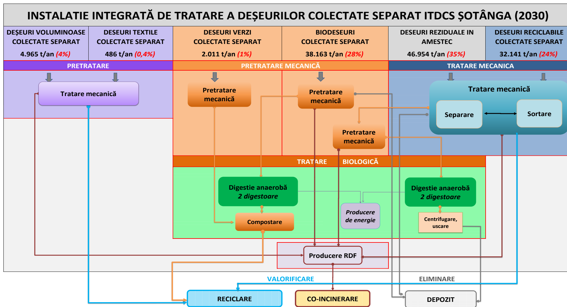
Figura 7-3: Fluxul deșeurilor în ITDCS Șotânga
