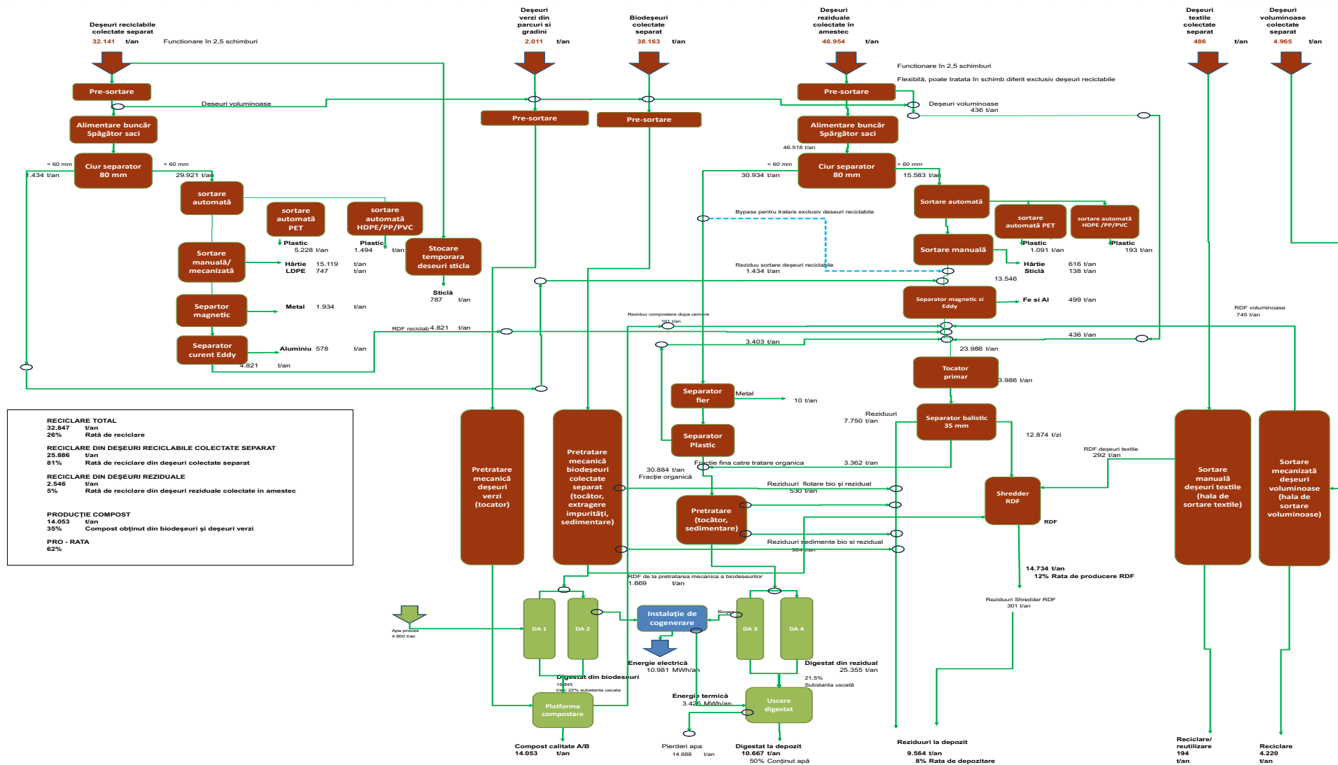
Figura 7-6: Schema Fluxului tehnologic în ITDCS Șotânga
