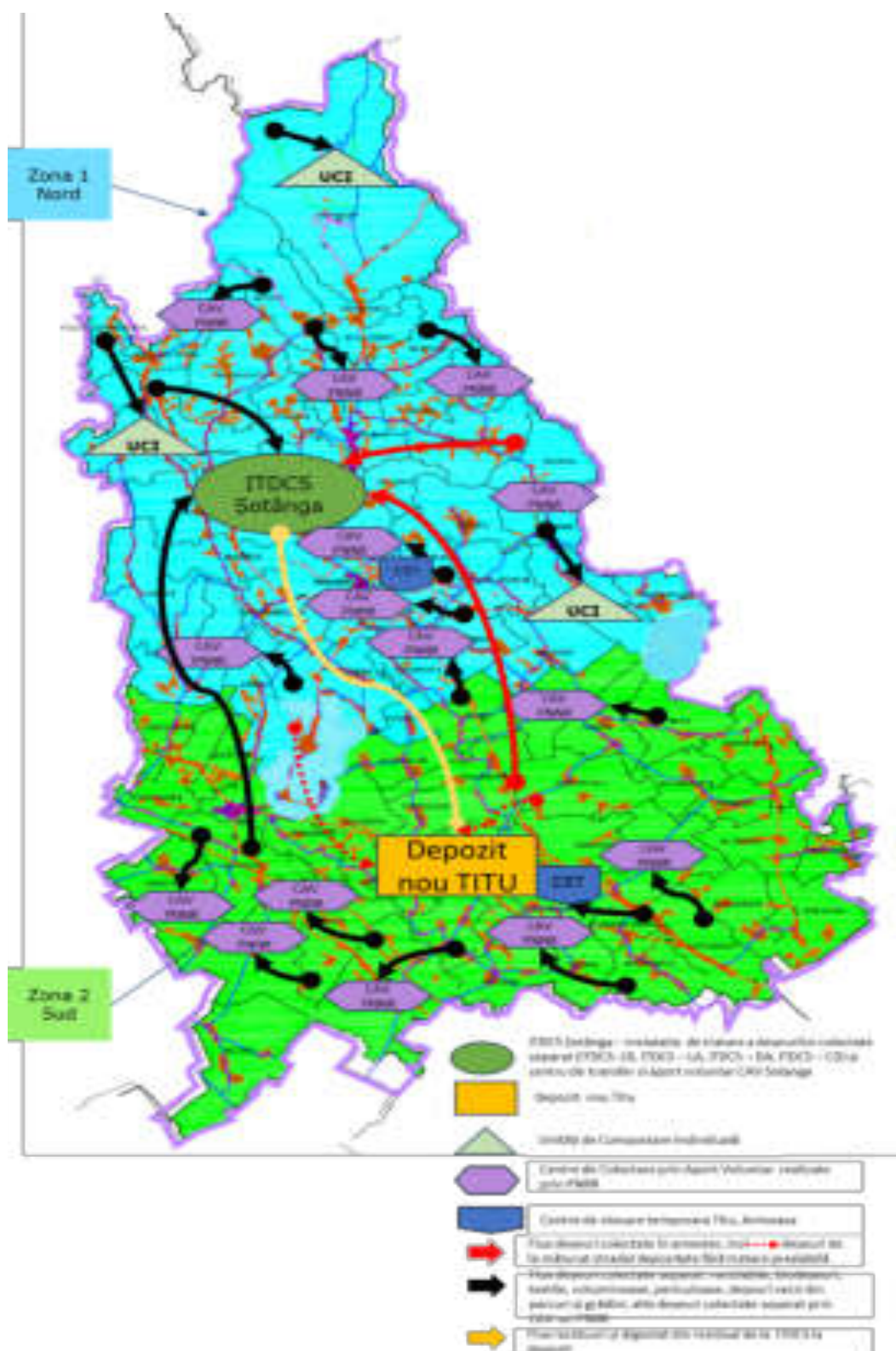
Figura 1-3: Fluxul generat al deșeurilor în cadrul SMID Dâmbovița începând cu anul 2030
